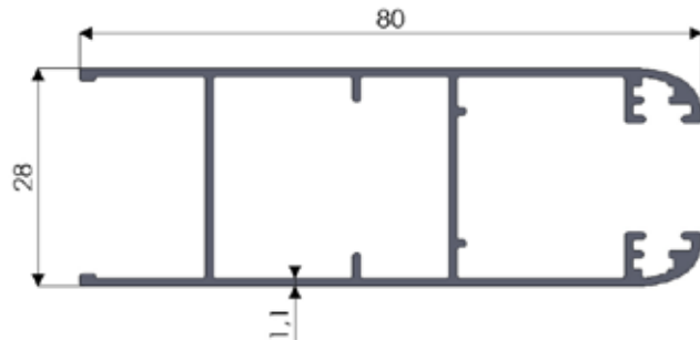
No: 1427 0,774 kg/m
