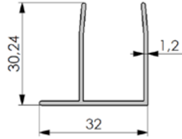
No: 1106 0,292 kg/m
