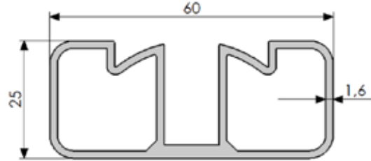
No: 1041 0,916 kg/m
