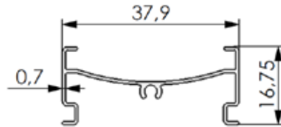
No: 1257 0,176 kg/m
