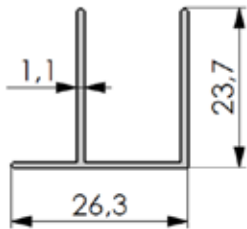
No: 1103 0,193 kg/m
