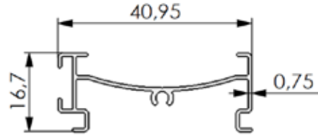
No: 1255 0,210 kg/m
