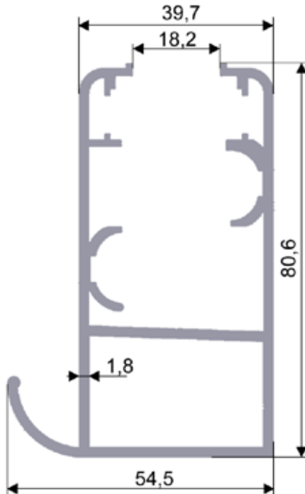
No: 1070 1,575 kg/m
