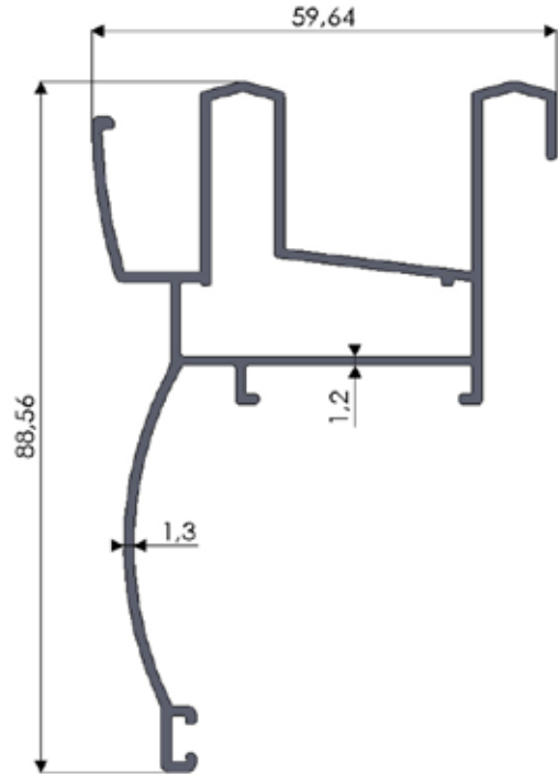
No: 1415 1,001 kg/m
