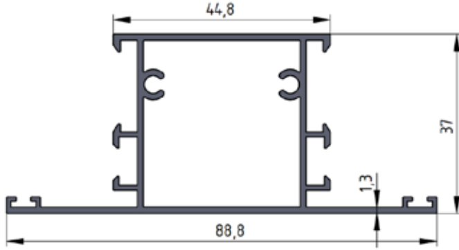
No: 1449 0,900 kg/m
