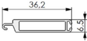
No: 1215 0,221 kg/m
