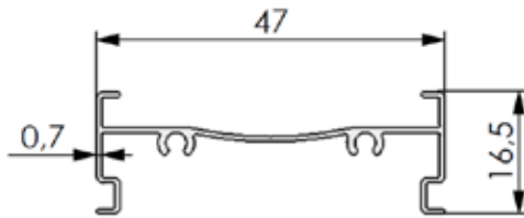
No: 1256 0,211 kg/m
