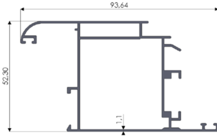
No: 1432 1,130 kg/m
