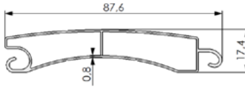
No: 1210 0,516 kg/m
