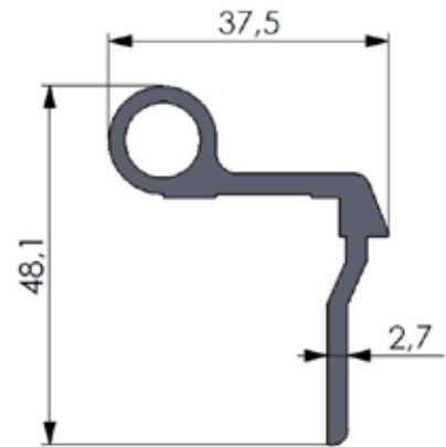
No: 1367 0,707 kg/m
