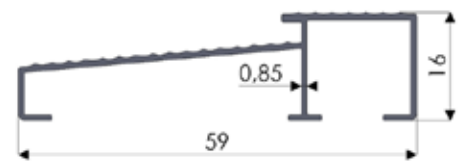
No: 1372 0,274 kg/m
