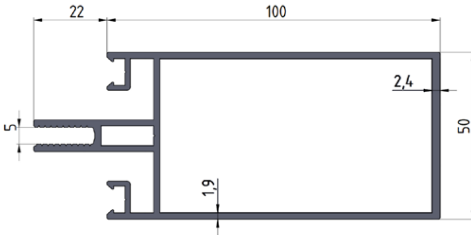
No: 1602 2,120 kg/m
