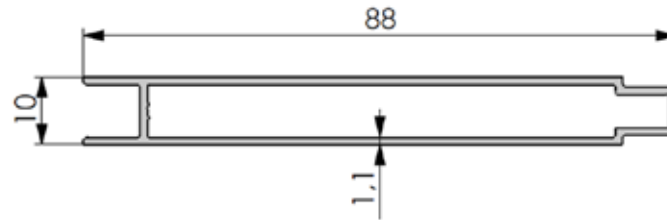
No: 1015 0,572 kg/m
