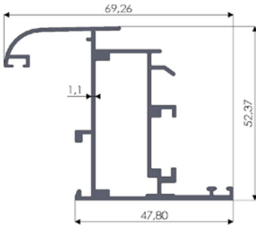
No: 1435 0,912 kg/m
