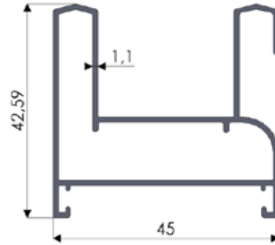
No: 1430 0,640 kg/m
