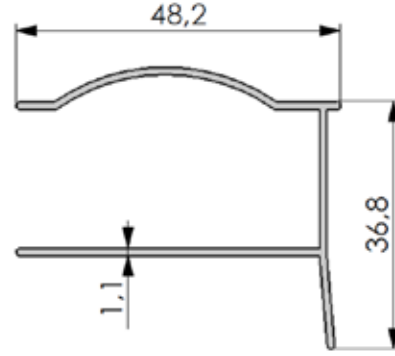
No: 1122 0,390 kg/m
