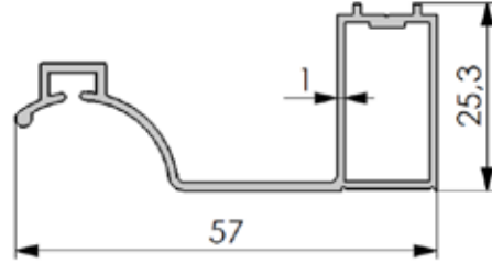
No: 1100 0,408 kg/m
