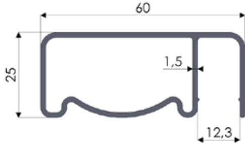
No: 1046 0,718 kg/m
