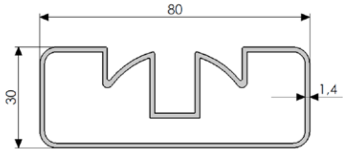
No: 1042 1,028 kg/m
