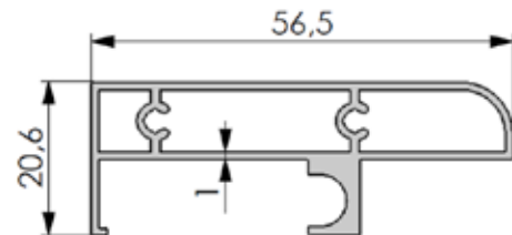
No: 1114 0,559 kg/m
