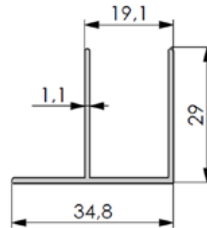
No: 1120 0,270 kg/m
