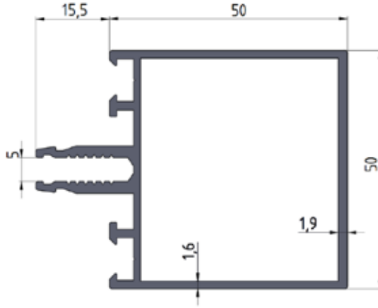
No: 1600 1,200 kg/m
