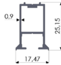
No: 1128 0,231 kg/m
