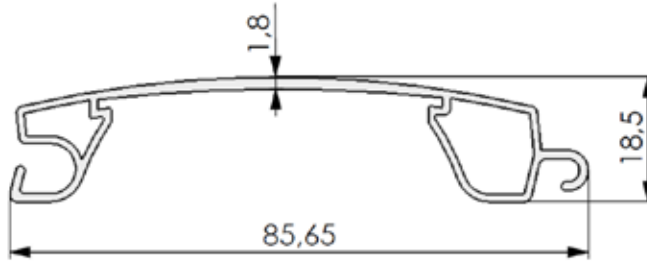
No: 1206 0,600 kg/m
