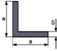
EQUAL ANGLES EŞKENAR
