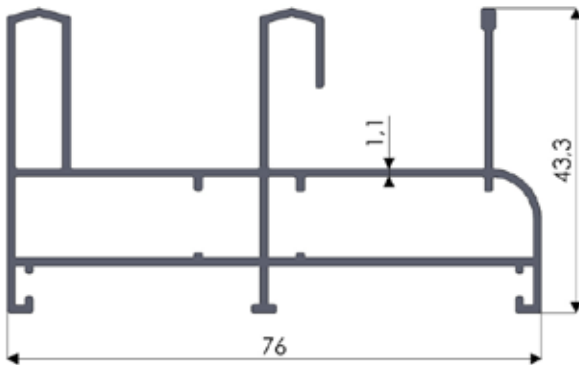
No: 1433 1,014 kg/m
