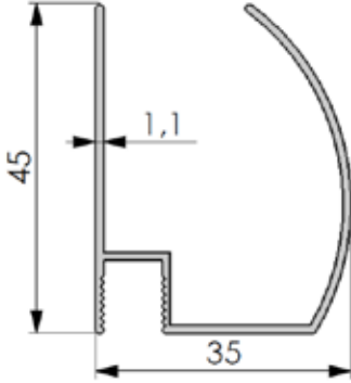
No: 1105 0,391 kg/m
